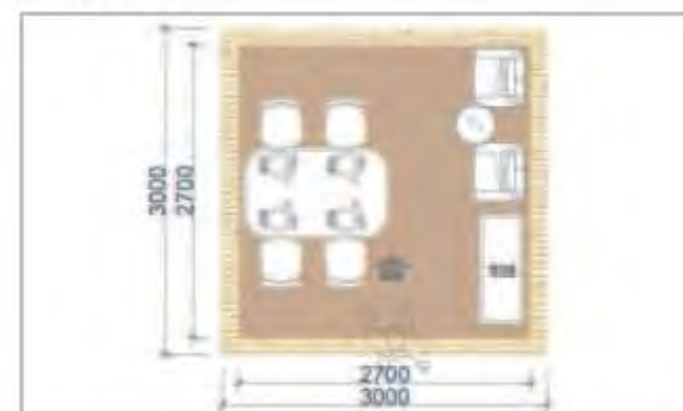
Q3 Tent Interior Plan Q3帐篷 室内平面图
